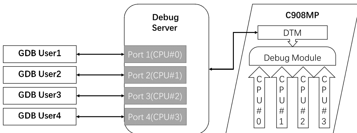
图 8.22: C908MP 多核多端口模型图
