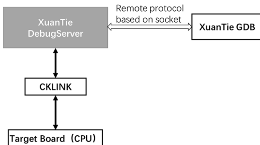
图 1.1: XuanTieDebugServer-Server 通信方式
