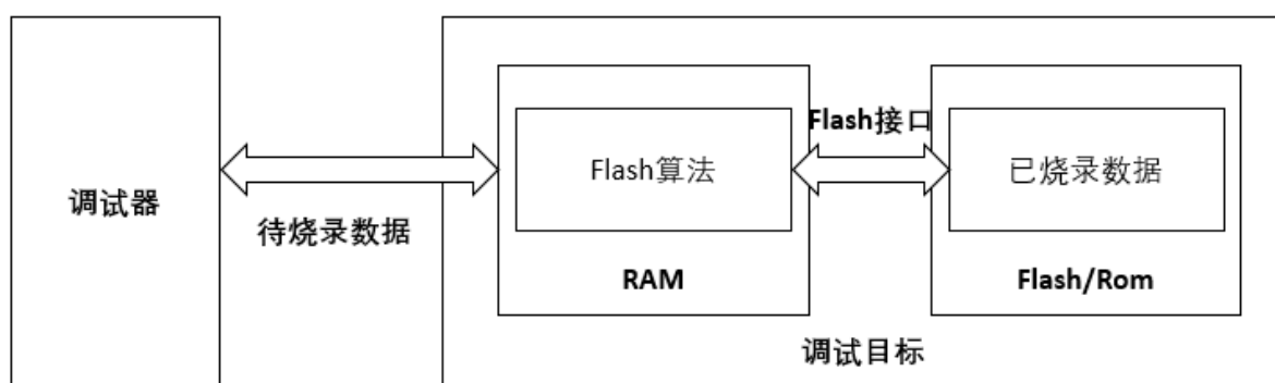
图 9.1: 调试器烧录 Flash 图示
