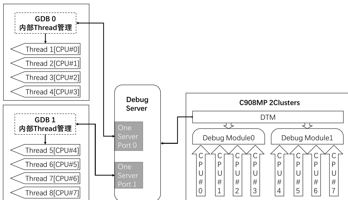
图 8.9: C908MP 多核多 Clusters 默认模型图
