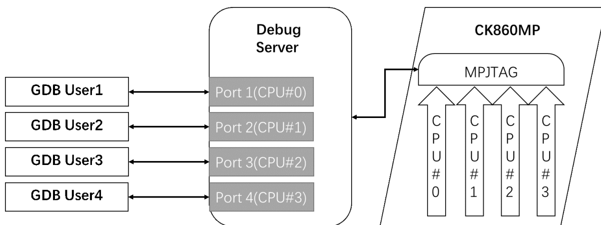
图 8.21: CK860MP 多核多端口模型图
