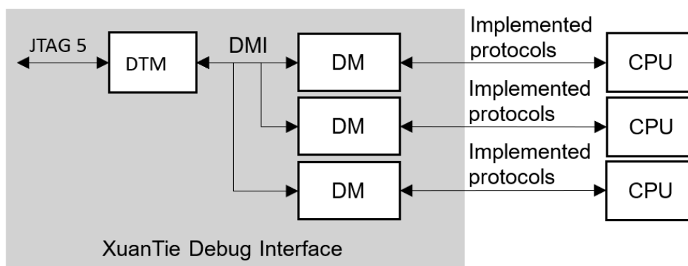
图 8.5: 多个 DM, 每个 DM 上挂一个 CPU
