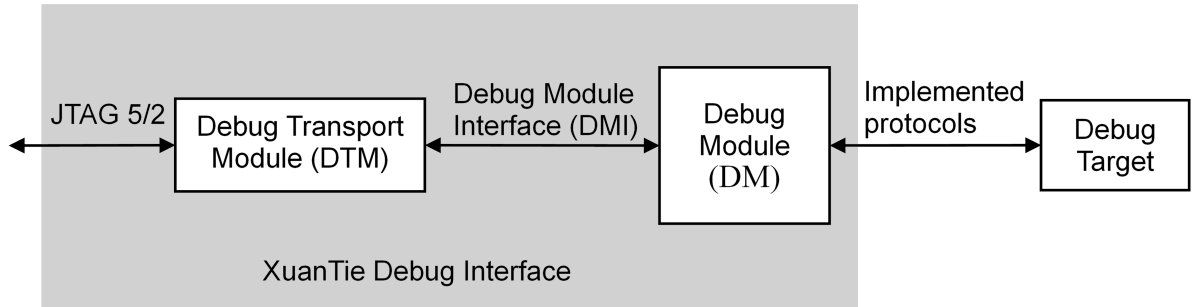
图 8.2: 多核调试整体框架
