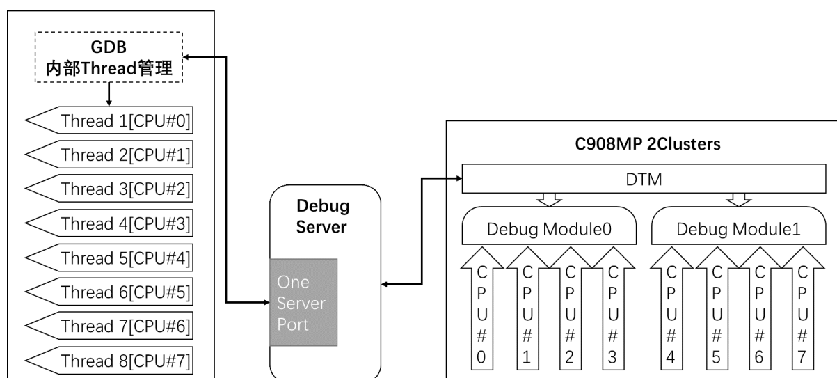
图 8.10: C908MP 多核多 Clusters -SMP 模型图
