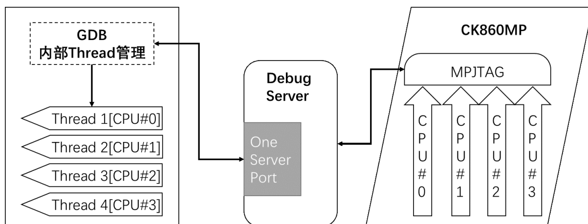
图 8.7: CK860MP 多核单端口模型图
