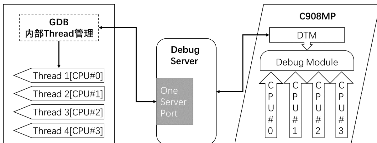
图 8.8: C908MP 多核单端口模型图
