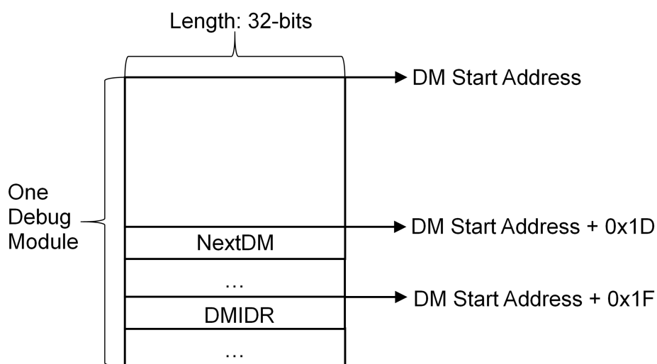
图 8.3: DM 单个 DM 布局
