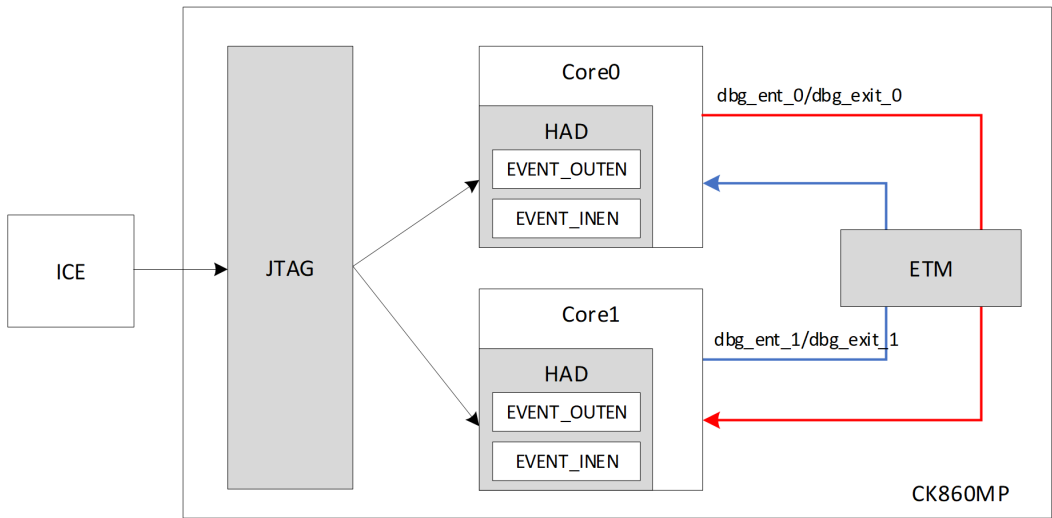
图 8.1: 多核调试整体框架
