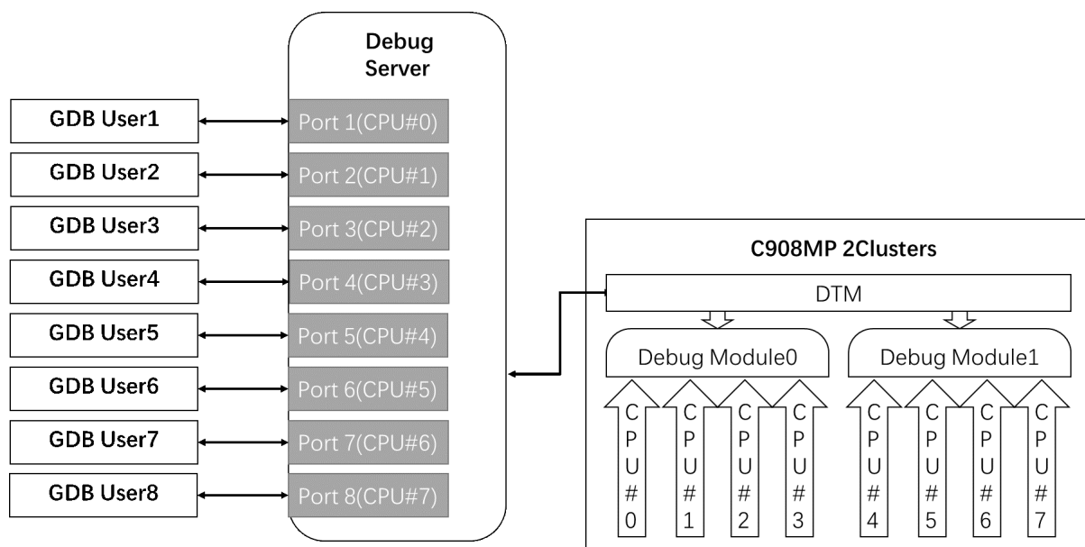
图 8.23: C908MP 多核多 Clusters 多端口模型图
