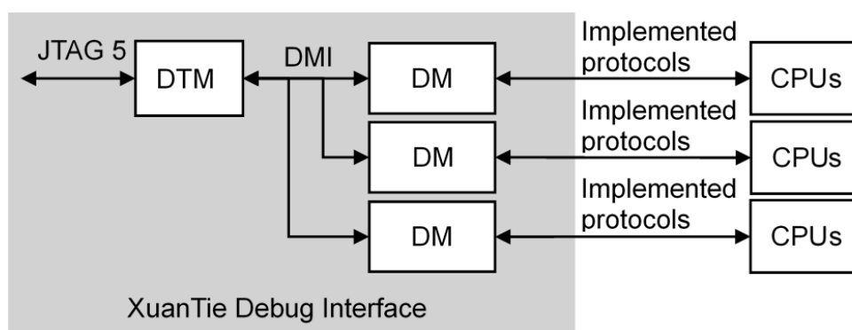
图 8.6: 多个 DMs, 每个 DM 上挂多个核
